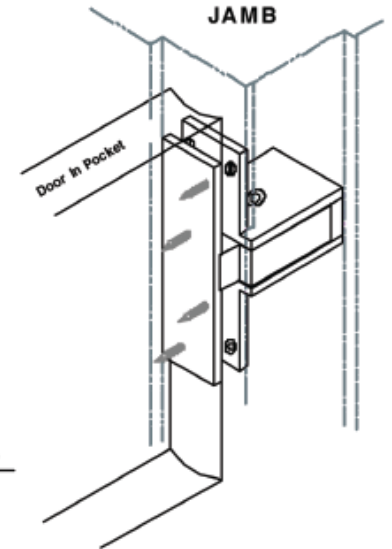
Door Jamb
