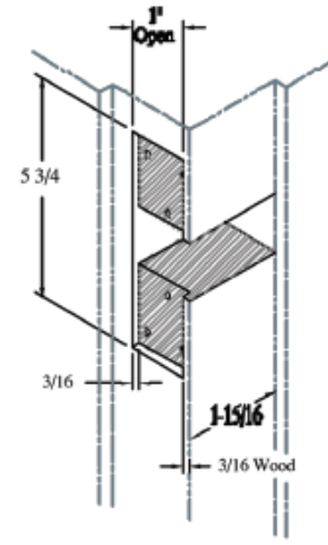
Door Jamb
