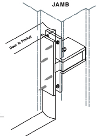
Door Jamb
