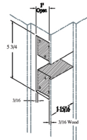
Door Jamb
