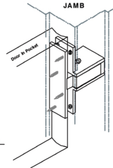
Door Jamb
