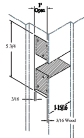
Door Jamb
