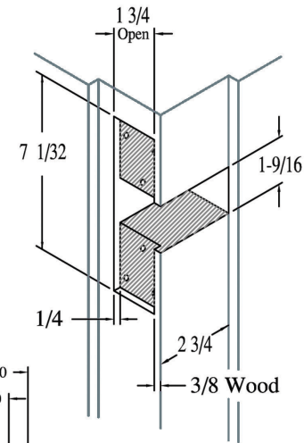
DOOR JAMB
