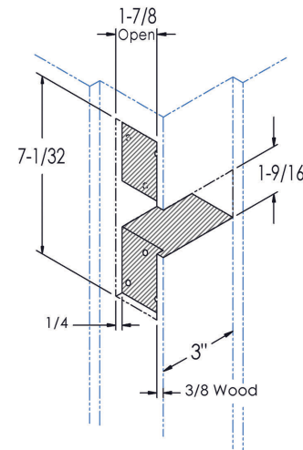
Door Jamb
