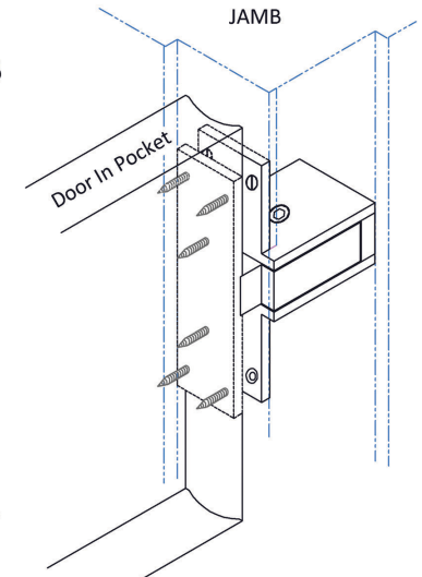
Door Jamb
