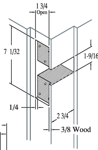
DOOR JAMB
