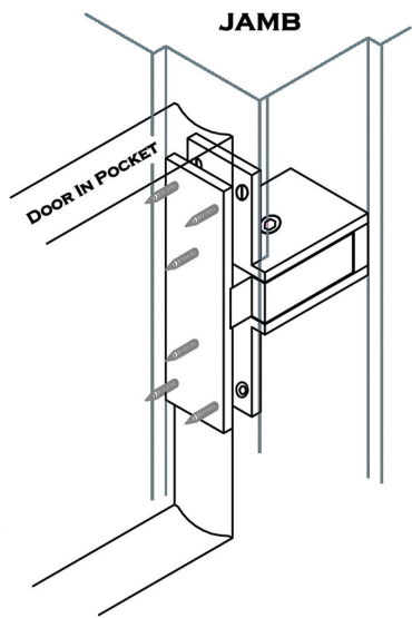
DOOR JAMB
